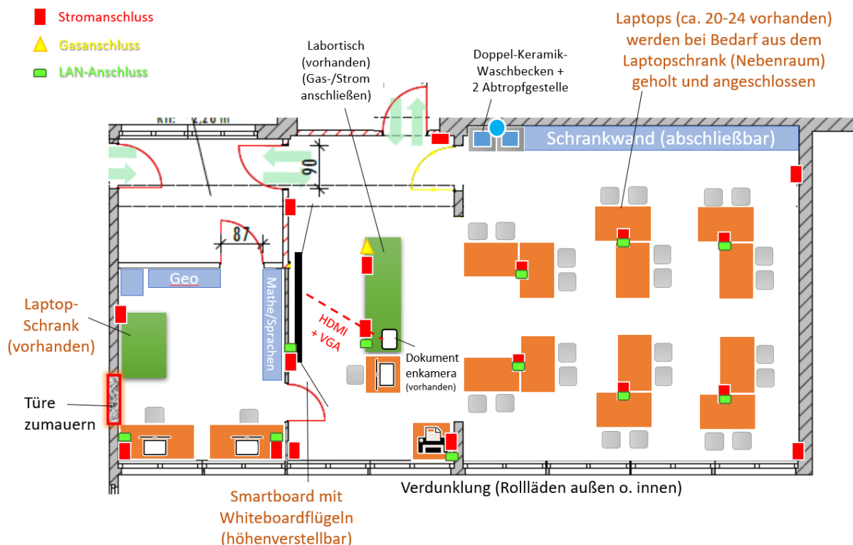
Abbildung 28 Grundriss des geplanten Computerlabors
